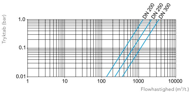
Typisk tryktabskurve, WPHD
